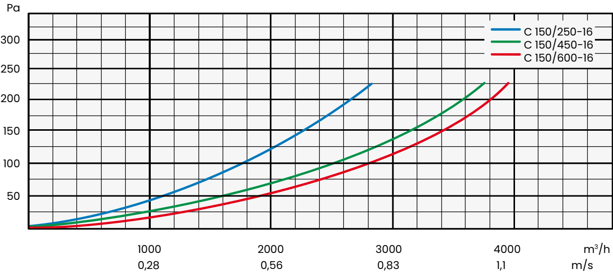
Courbe de débit d'air pour le filtre à charbon UltraSorb C150
