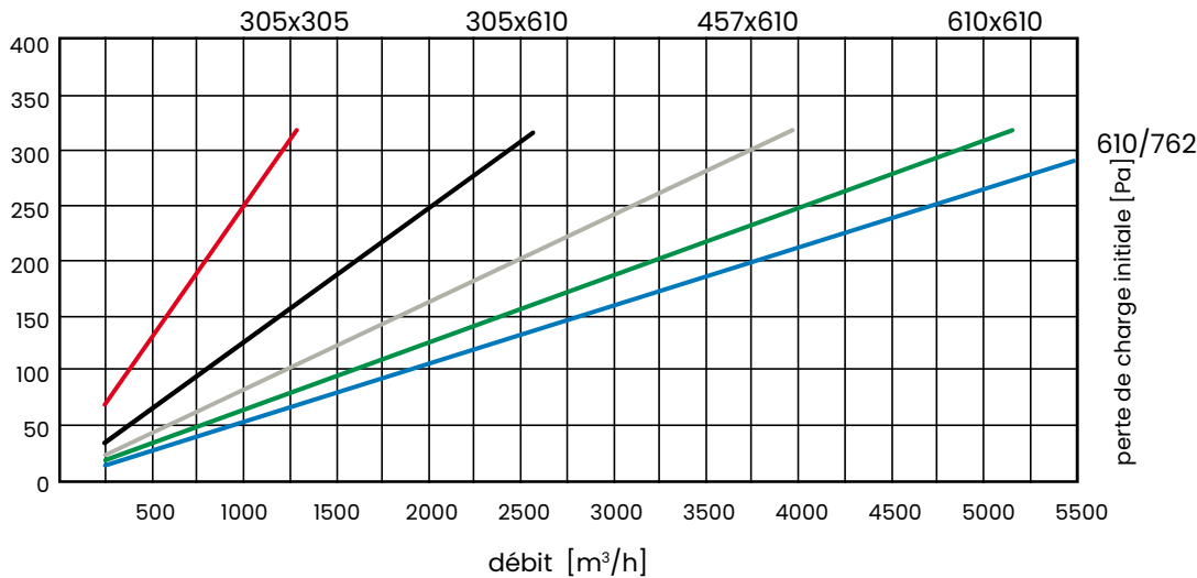
Graphique de la perte de charge des filtres en classe H13 avec surface de filtration augmentée
