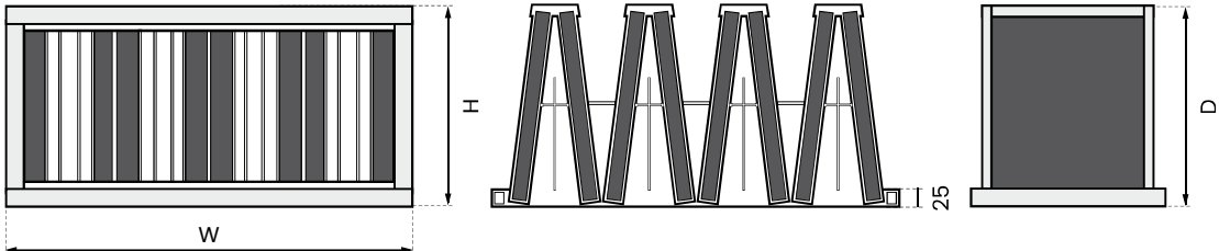
Données techniques pour différents modèles de filtres UltraKomp V440
