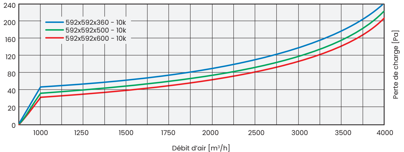
Pertes de charge en fonction du débit pour les filtres UltraTec 9
