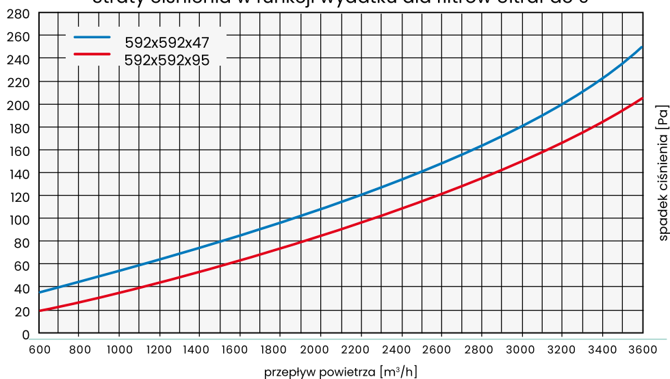
Straty ciśnienia w funkcji wydátku dla filtrów UltraPac 9
