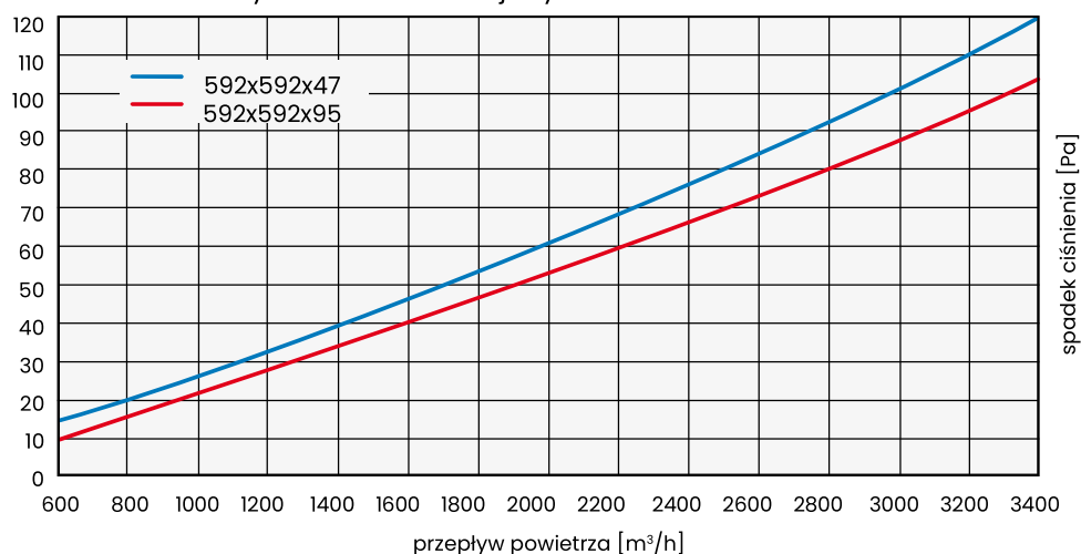
Straty ciśnienia w funkcji wydátku dla filtrów UltraPac 7
