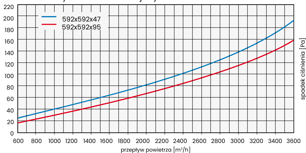
Straty ciśnienia w funkcji wydátku dla filtrów UltraPac 8
